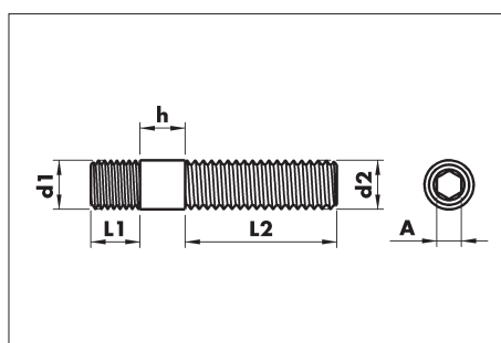
Bolt
