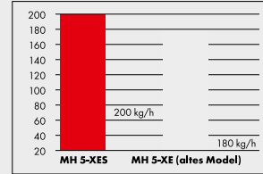
Meißelleistung in kg/h (Material Beton B 35)
